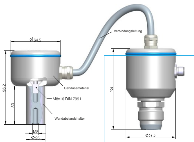
Beispielsensor für die Montage des DES z. B. SLI03, SDT03, STS...
